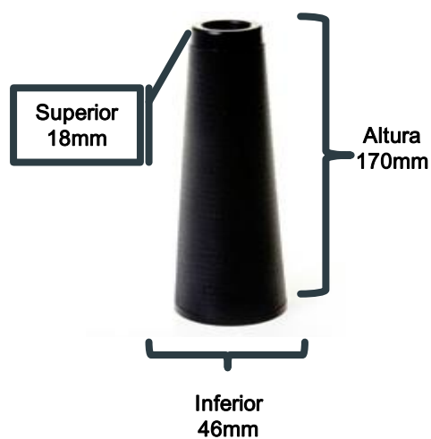
Conical 3/30 - conicidade 3°30
