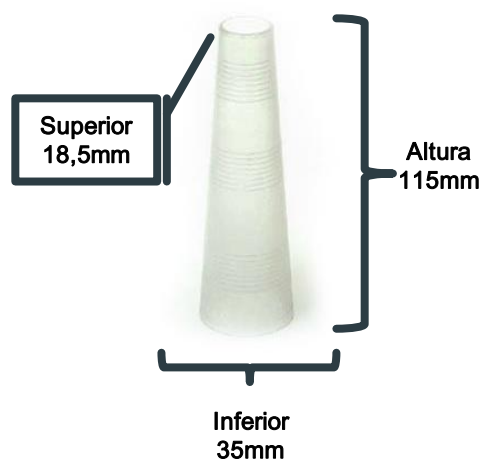
Conical 4°20- conicidade 4°
