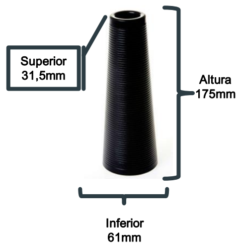
Conical 175 - conicidade 3°30
