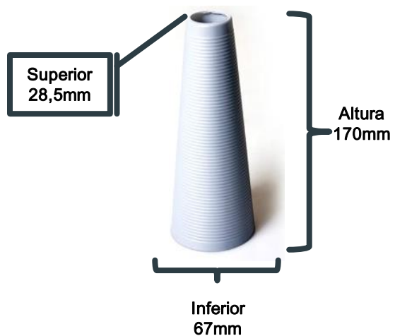
Conical 5/57 - conicidade 5.57°
